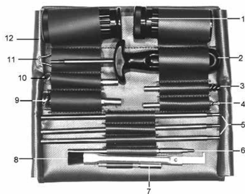
Abbildung 13: Putzzeug
