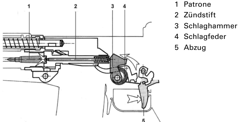
Abbildung 15: Schussauslösung
